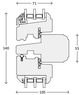
waagerechter Pfosten
