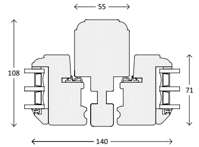
senkrechter Pfosten
