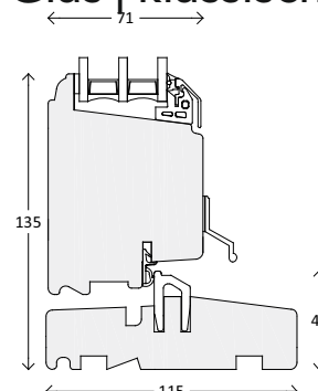
unten Hartholzschwelle
