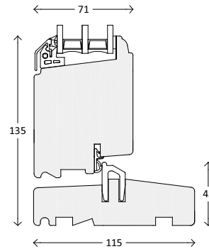
unten Hartholzschwelle
