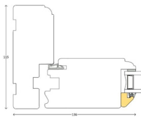
oben und unten auswärts öffnend (bsp. Hartholzschwelle)
